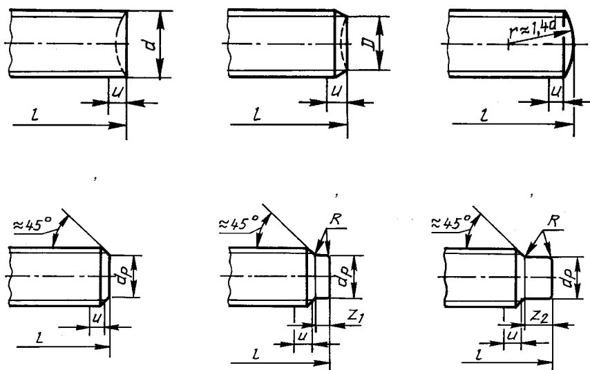
Ступенчатый конец с конусом
