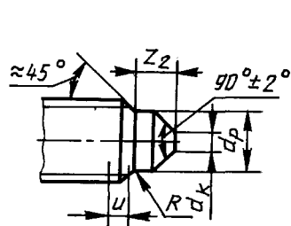
Ступенчатый конец с конусом
